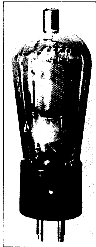
Fig. 18 - Radiotron UX-222.
